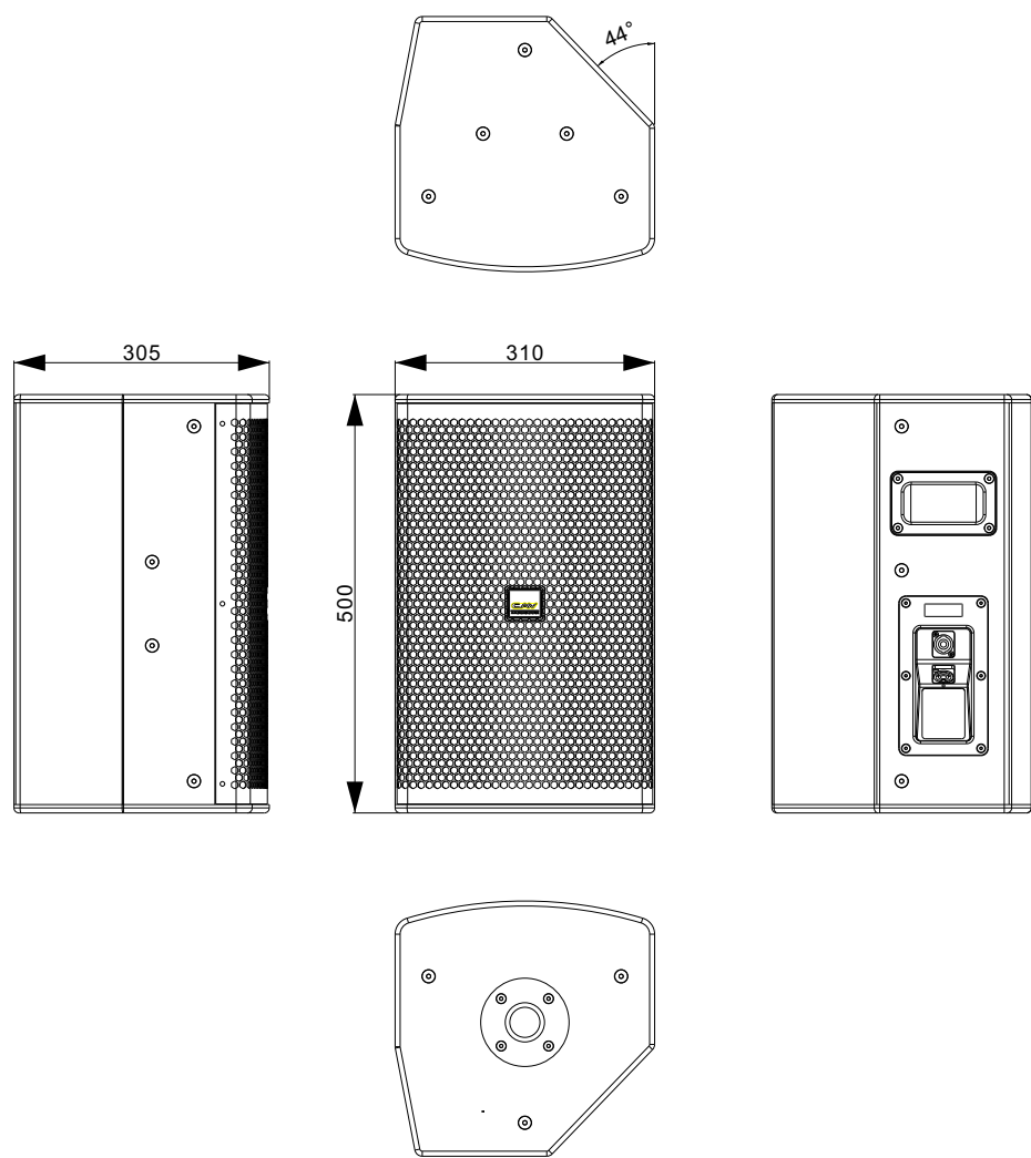
外形尺寸示意图：
